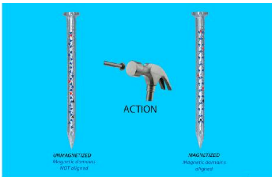
Fig 1: Het magnetiseringsproces van ijzer.
