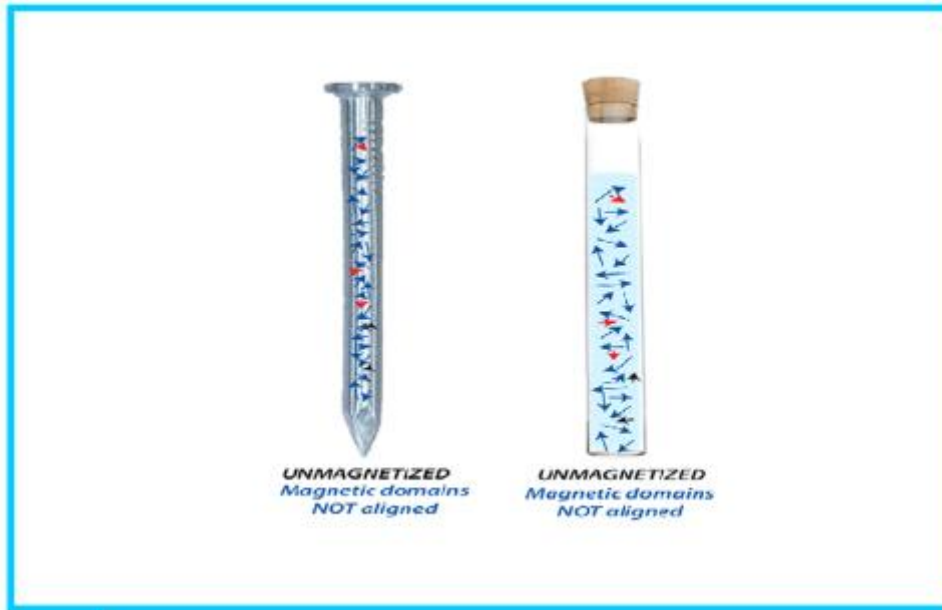
Fig 2: De overeenkomst van de atomische structuren van de twee magnetische stoffen op aarde voor hergroepering van hun elektronen.
