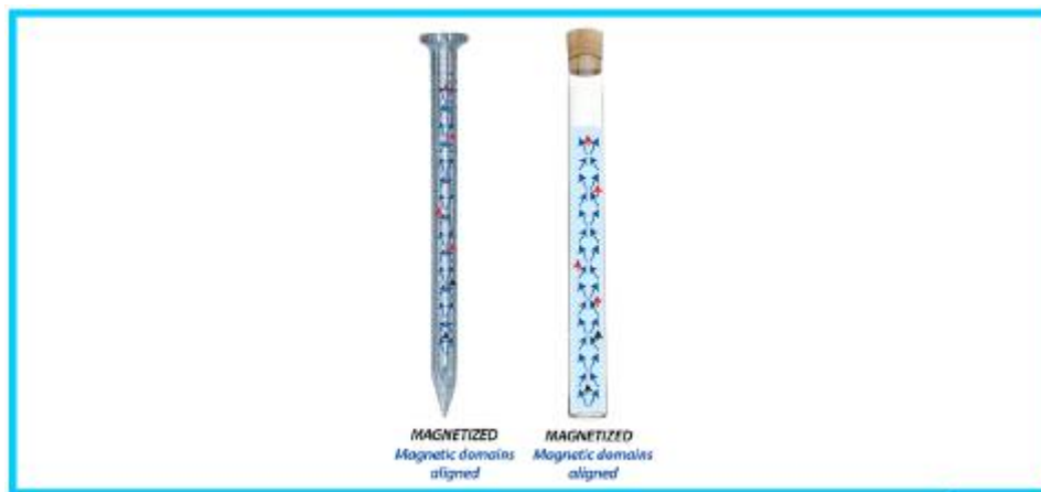
Fig 4: Het gemagnetiseerd ijzer, wateratomen en zuurstofmoleculen.
